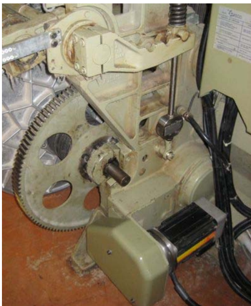
SVOLGITORE DI ORDITO telaio TP600
